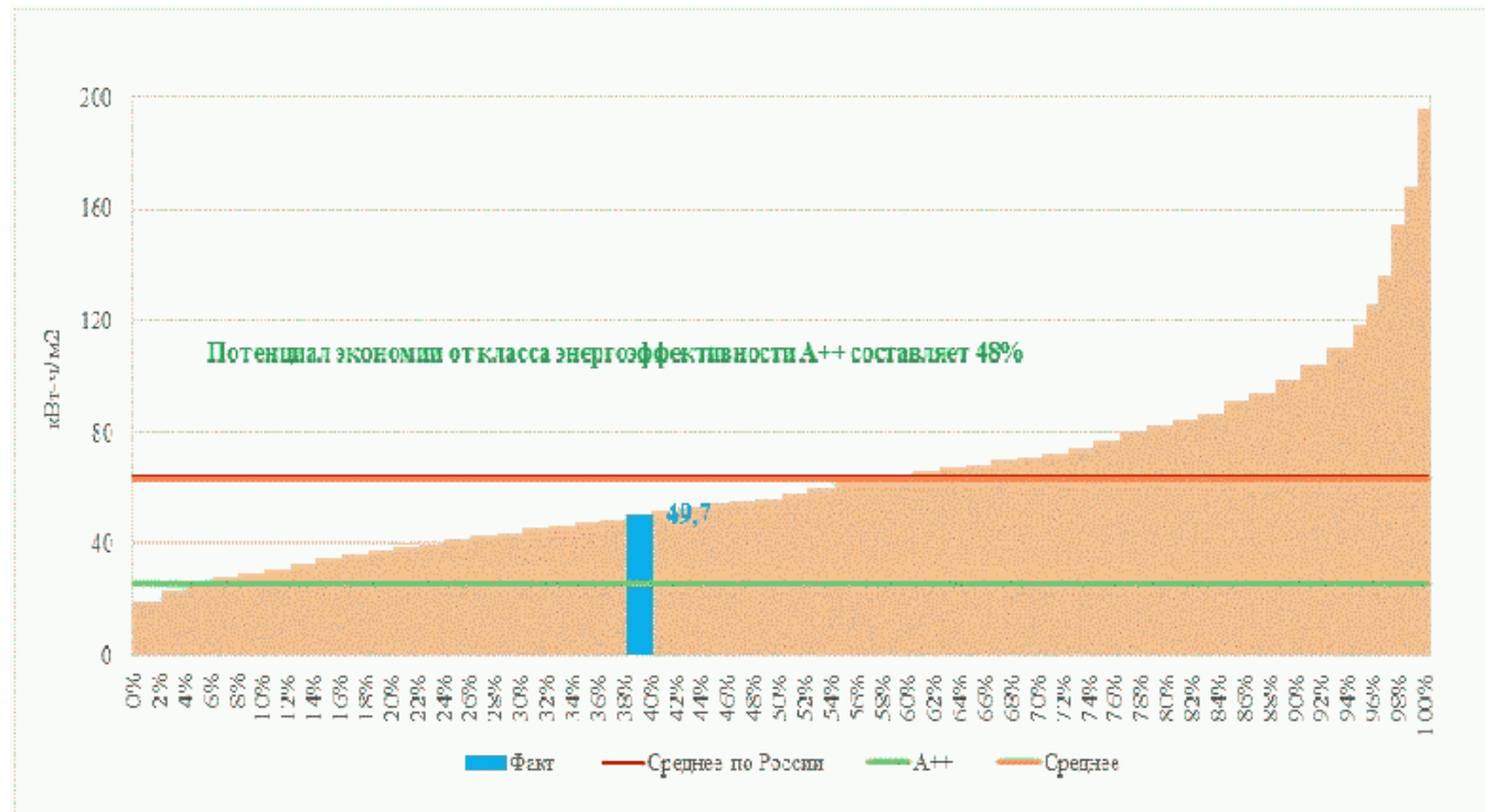
Рисунок 2. Типовая кривая распределения удельного расхода тепловой энергии на цели горячего водоснабжения
